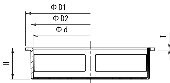
断面 A-A
